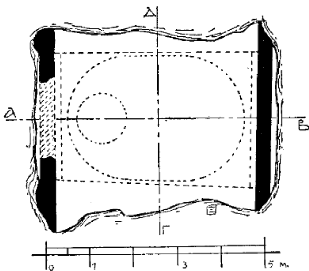
Εἰκ. 6. Φρέαρ παρὰ τὸν Προφήτην Ἑλὶαν (κάτοψις καὶ τομαί).
