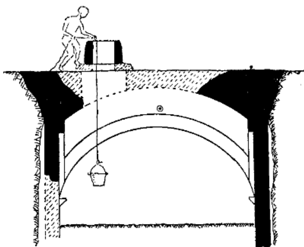
ΤΟΜΗ Α-Β
