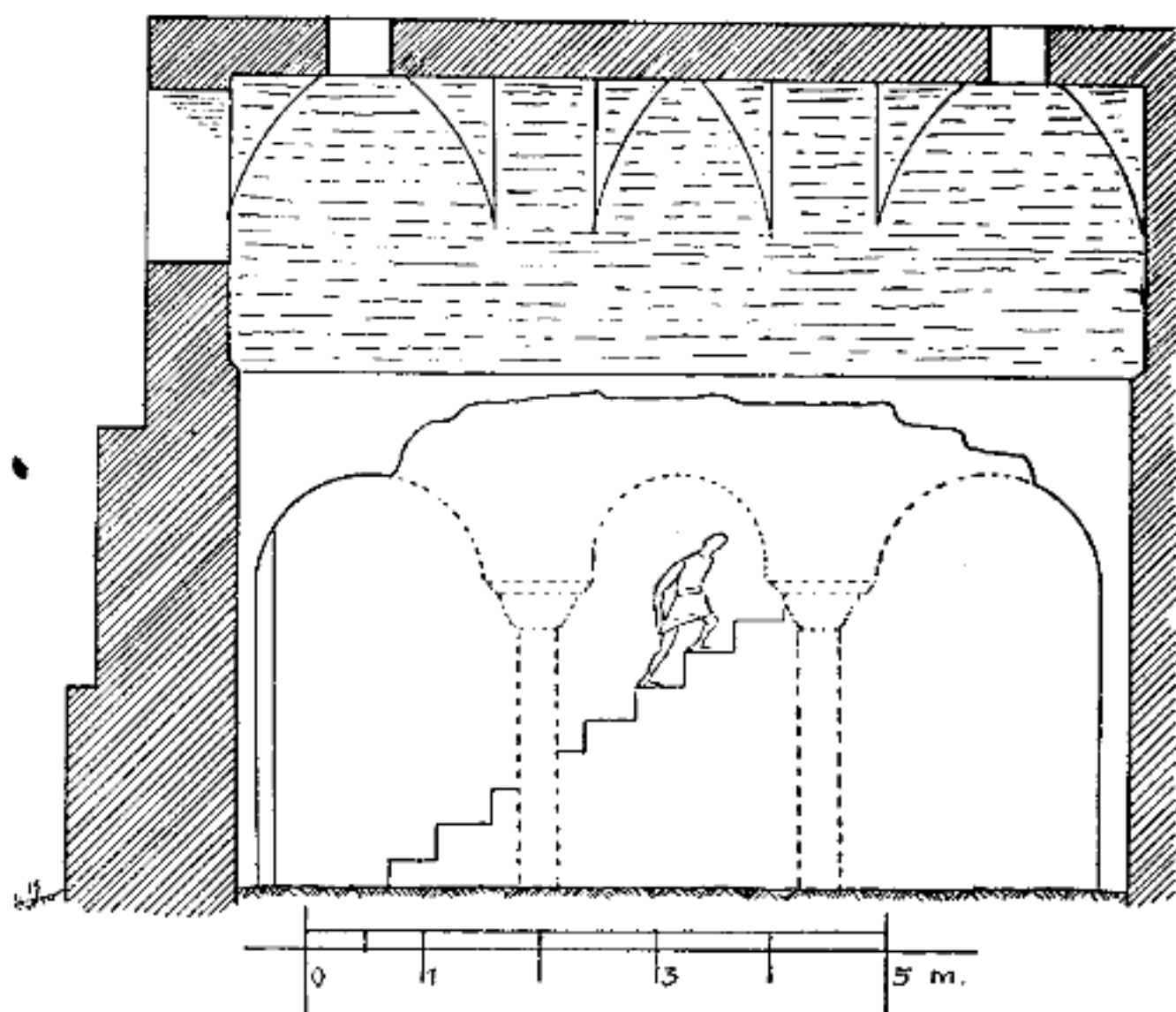
Εἰκ. 3. Τομὴ κατὰ πλάτος.
