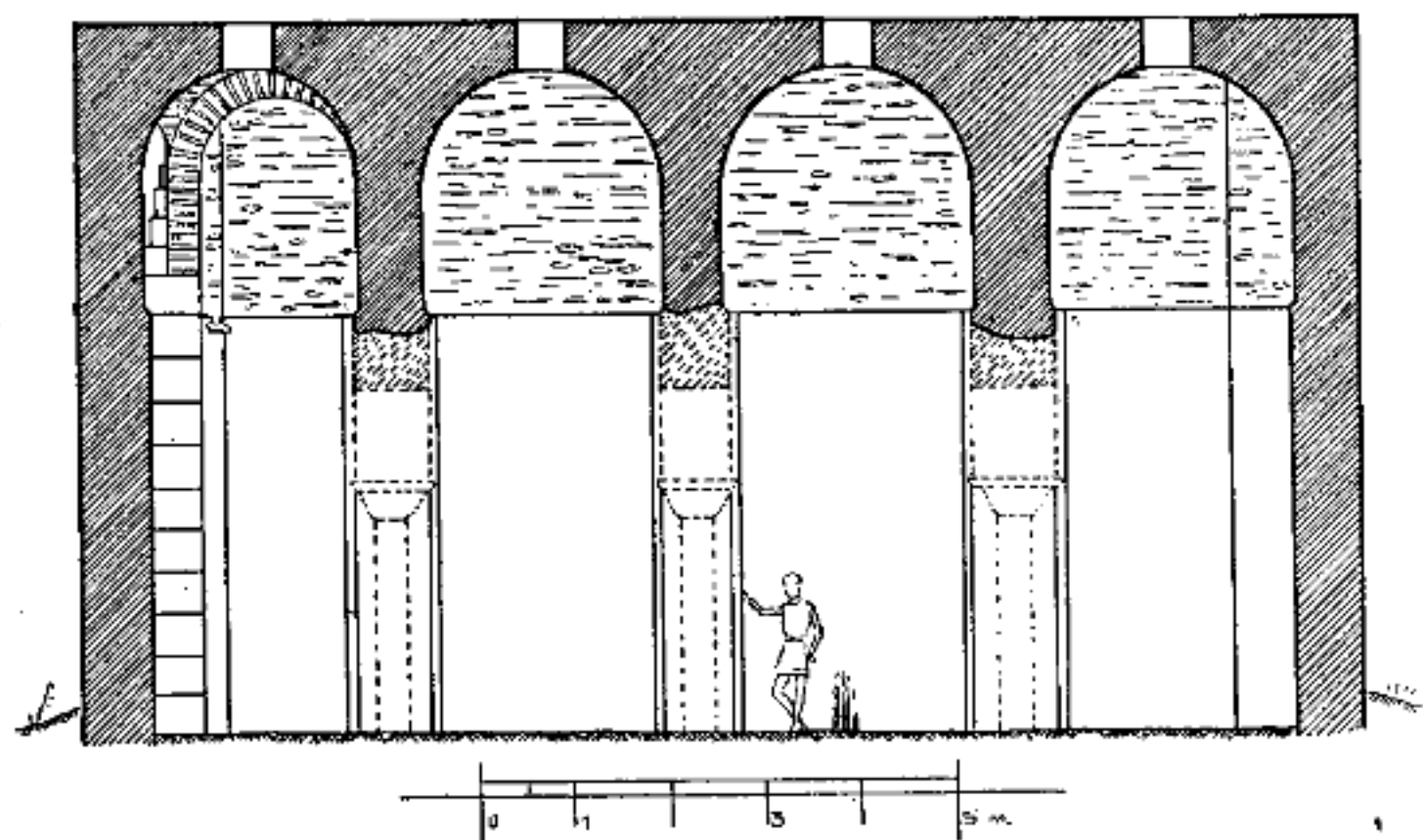
Εἰκ. 2. Τομή τῆς κινστήριας κατὰ μῆκος.
