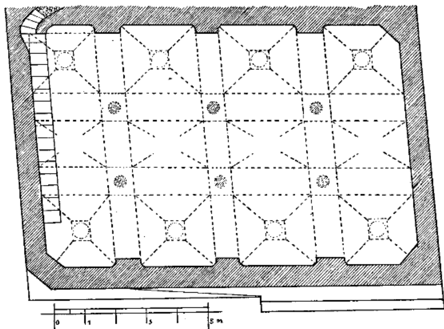
Εἰκ. 1. Κάτοψις τῆς κινστήριας.
