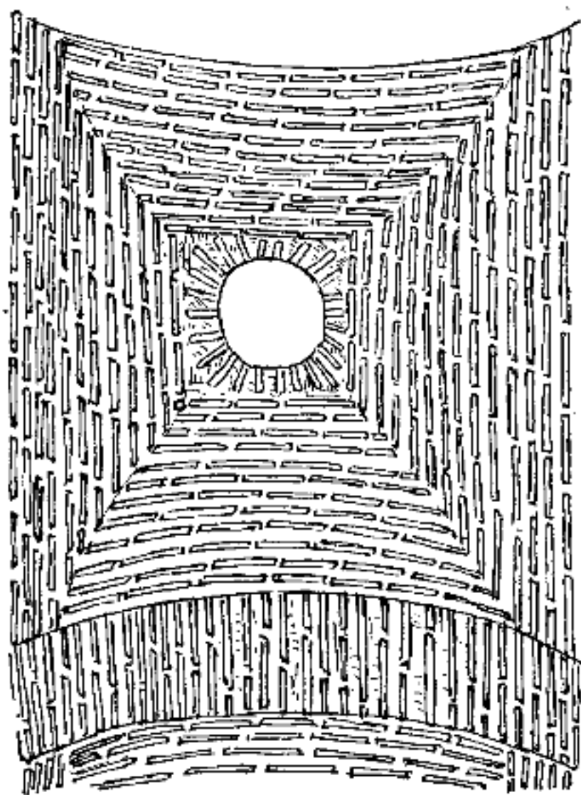
Εἰκ. 5. Λεπτομέρεια τῆς κατασκευῆς τῶν μοναστηριακῶν θόλων εἰς τὴν ὀροφήν τῆς δεξαμενῆς.
