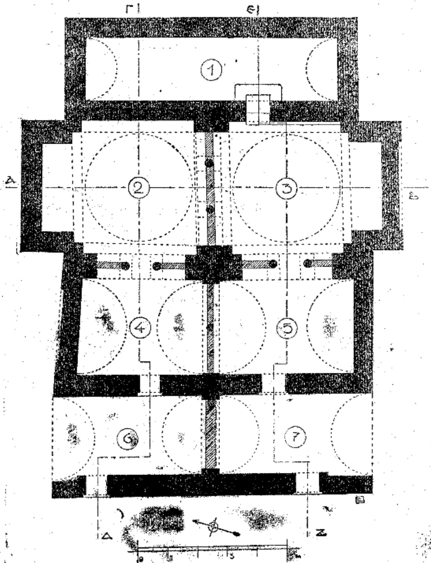
Εἰχ. 1.—Κάτοψις τοῦ λουτρῶνος [ὡς ἔχει σήμερον.
