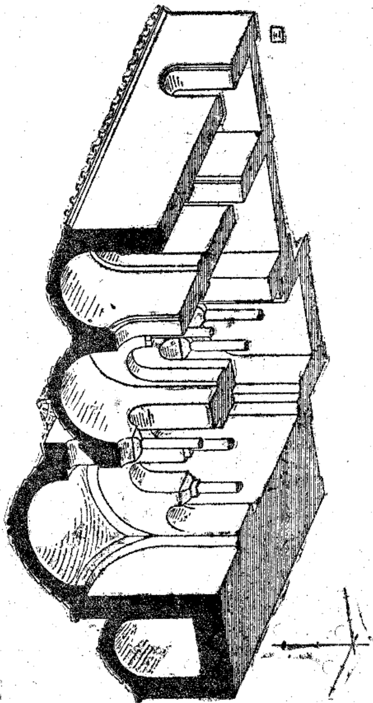
Εἰκ. 7.—Τομή ἰσομετρικῆ δεικνύουσα τὴν ἑσπερικὴν διαρρύθμισιν τοῦ λουτροῦ.
